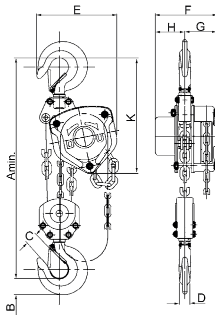
Model Silverline Stira S 3000 - 5000 kg, dvojprameňová reťaz
